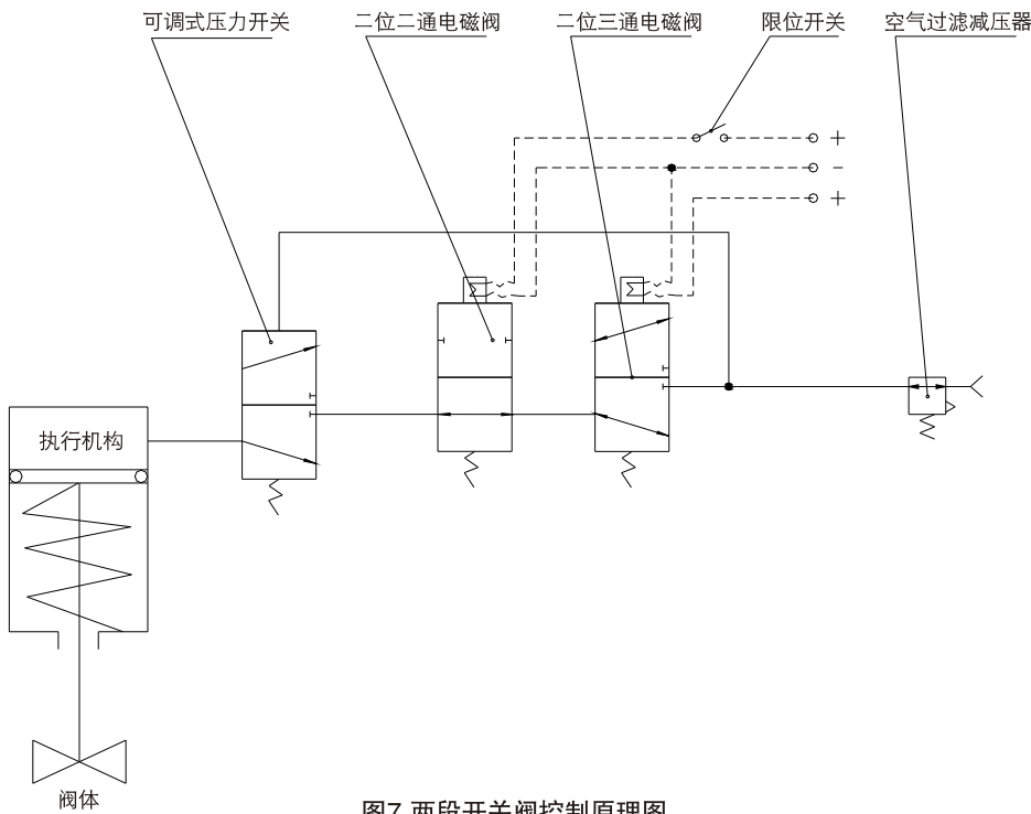
图7 两段开关阀控制原理图
