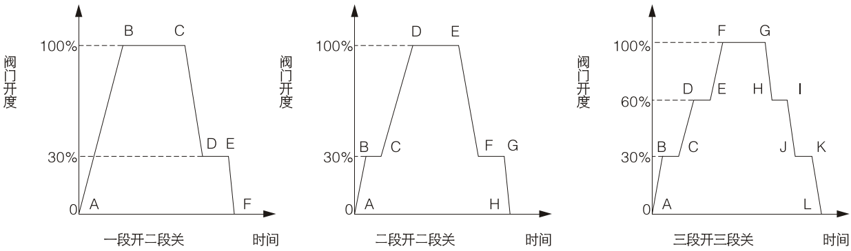
图2 流量开关特性曲线图
